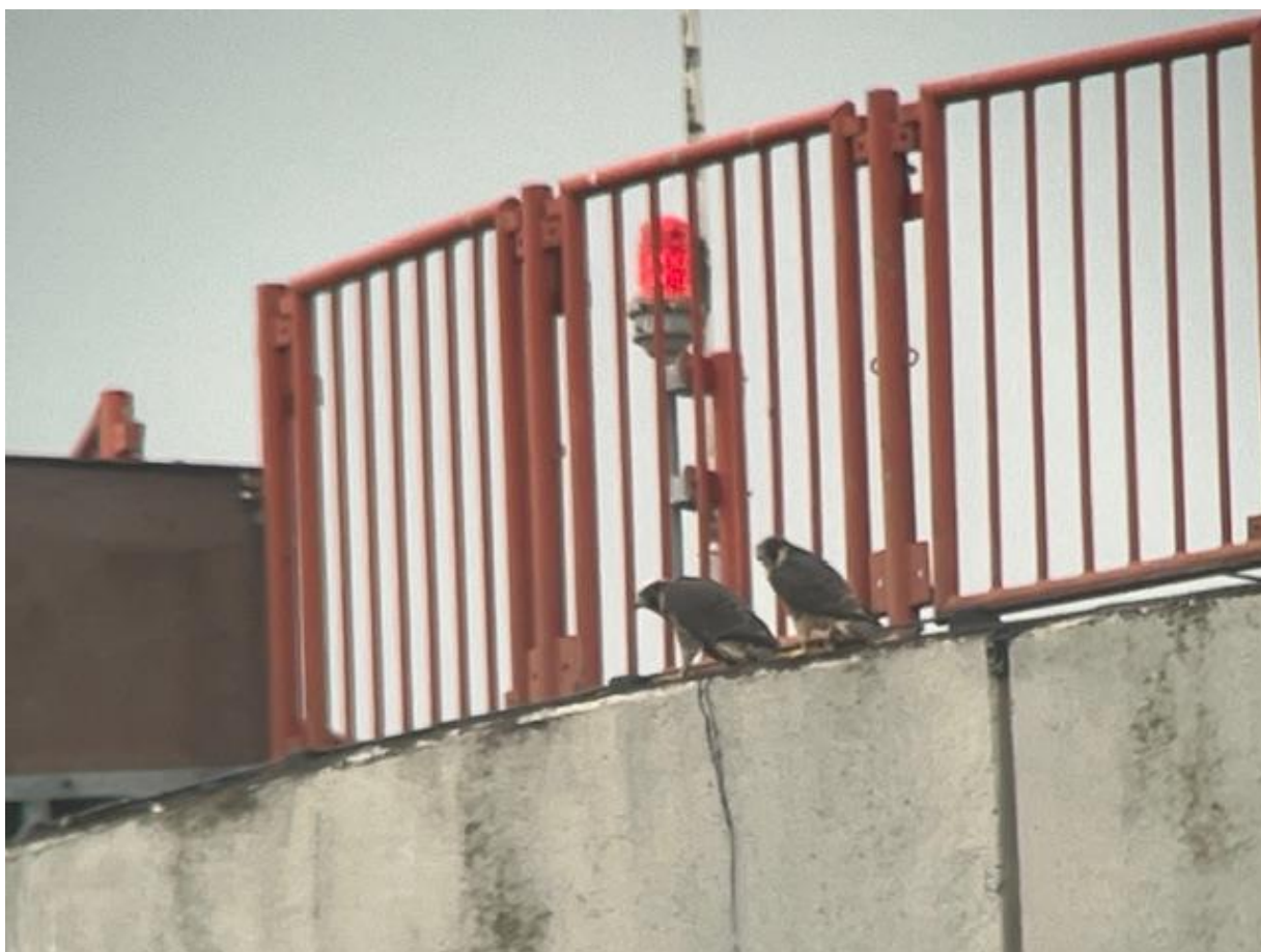
De Slechtvalk op de TV-toren in Goes is de laatste 7 jaar steeds aanwezig. Het broedsucces halveerde.
